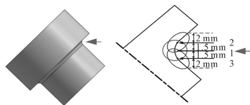
(a) 激光束入射方向和光斑搭接示意图
