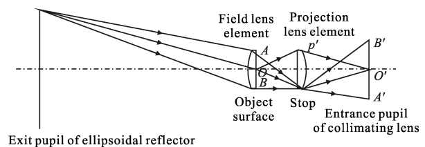
图 2 积分器的成像关系图
