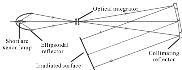
图 1 太阳模拟器工作原理
