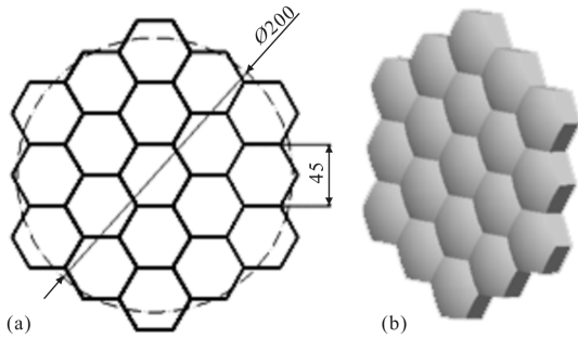
图 3 积分器排列示意图
