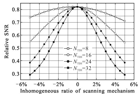
图 6 扫描非均匀性对不同 TDI 级数探测器的影响 Fig.6 Effect of scanning inhomogeneous on TDI levels
