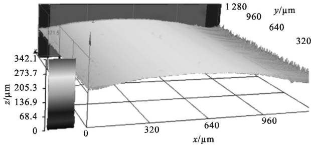
图 3 CaF 2 盘型腔的粗糙度测试图
