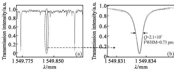
图 5 (a) CaF 2 盘腔谐振谱线; (b) 谐振谱线洛伦兹拟合曲线
