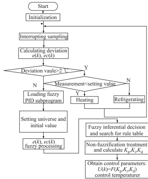
图 5 主程序流程
