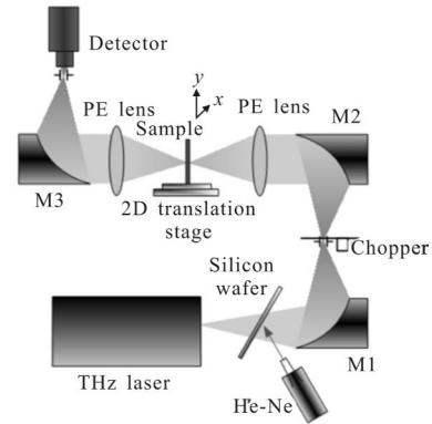
图 1 2.52 THz 共焦扫描成像实验装置
