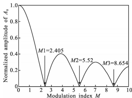
图 2 载波分量和调制系数的关系
