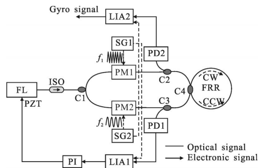
图 1 谐振式光纤陀螺系统工作原理图
