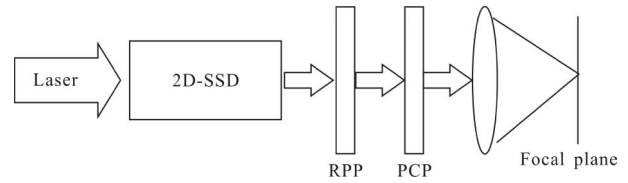
图1 单光束“二维 SSD+RPP+OPCP”的匀滑方案
