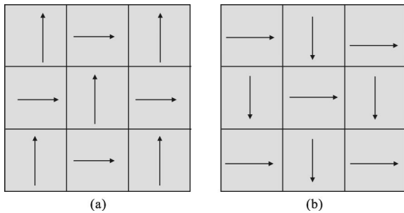
图 3 正交偏振板的互补组合
