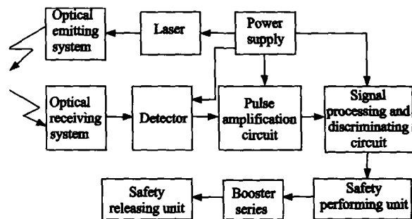
图1 激光引信原理框图
