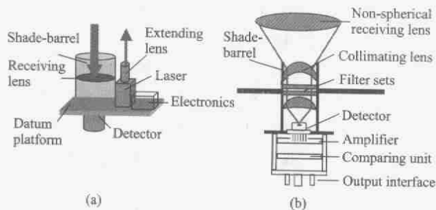
图 2 光学系统和接收光路结构图
