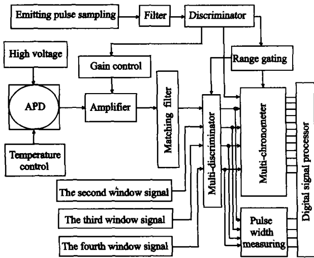
图 3 信号处理及电子学部件结构图
