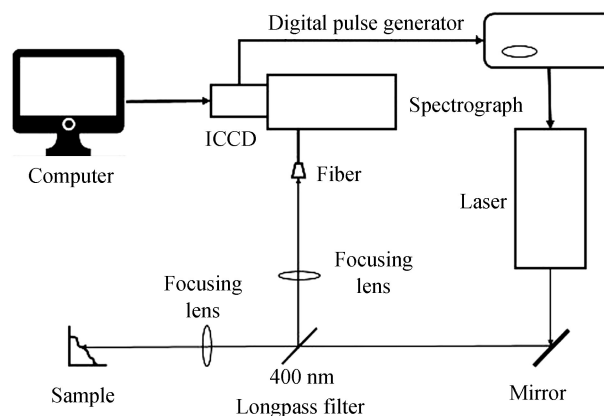
图 1 LIBS 实验系统图
