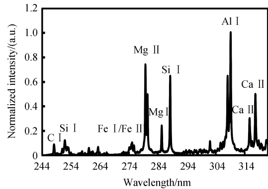
图 2 样品 6 的激光诱导击穿光谱图
