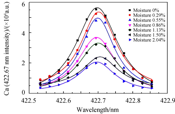
图 4 不同水分含量下 Ca 谱线 Lorentz 拟合
