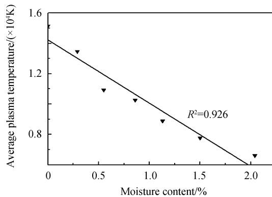
图 3 不同水分含量下等离子体温度及平均等离子体温度
