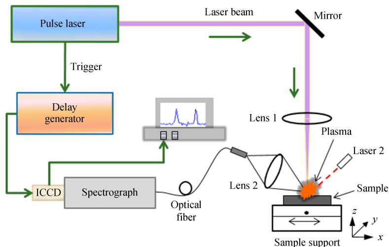
图 1 LIBS 分析系统装置示意图 Fig.1 Schematic diagram of LIBS analysis system
