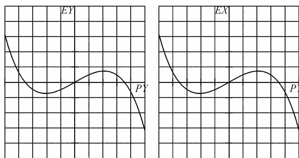
(b) Ray fan of spherical lens
