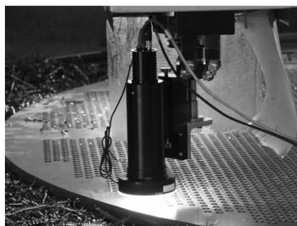
图 6 支撑板板孔精密测量系统
