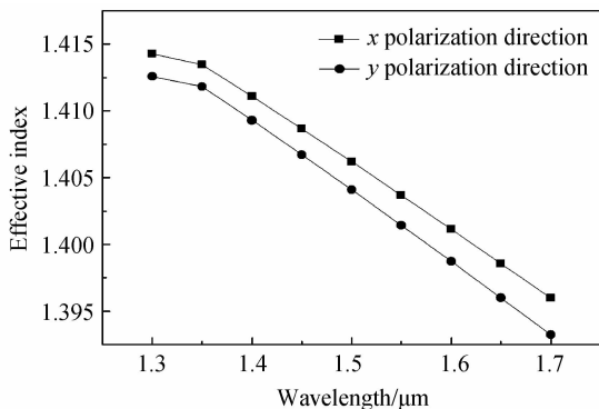
图 8 有效折射率随波长的变化
