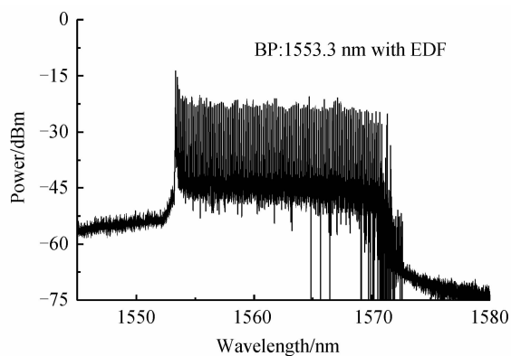
图 6 加入 EDF 后的光谱,OSA1 观测
