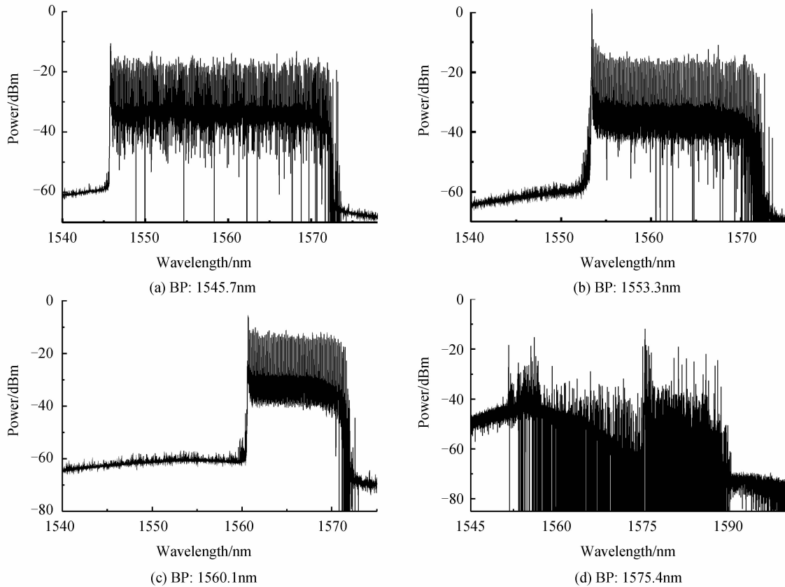
图3 BP波长对输出波长数影响, RP:800mW
