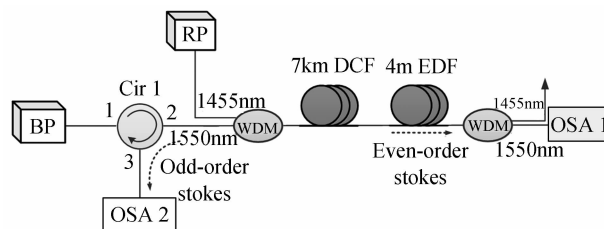
图 1 全开腔布里渊喇曼激光器结构原理图
