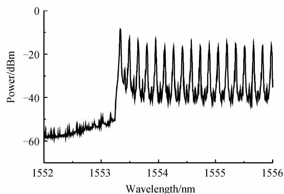
图 4 OSA1 观测输出光谱,RP:800 mW
