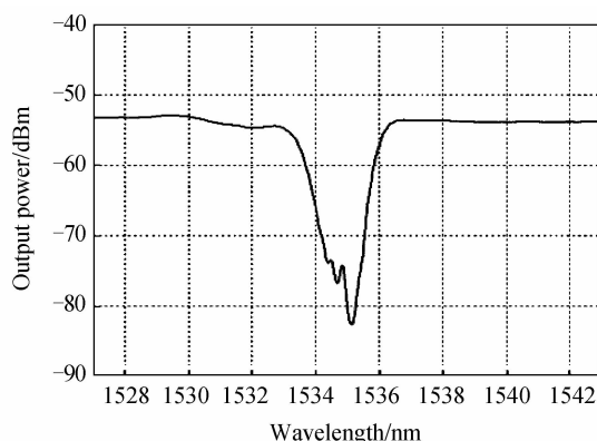
图 2 保偏光纤布喇格光栅透射谱
