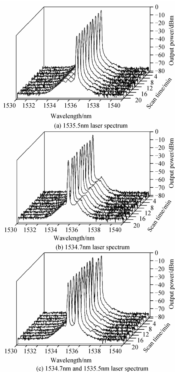
图6 输出激光光谱稳定性
