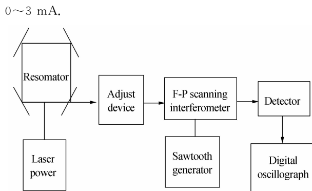
图 2 测试系统装置示意图
