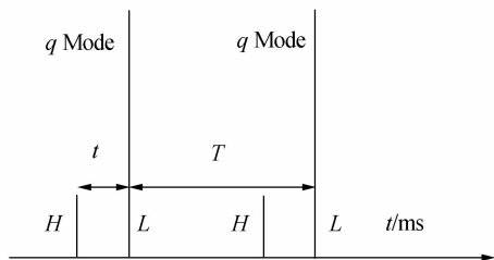
图3 脉冲信号示意图
