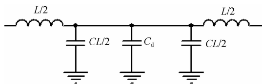
图5 微带线的电容与电感和光电二极管的结电容组成的等效电路
