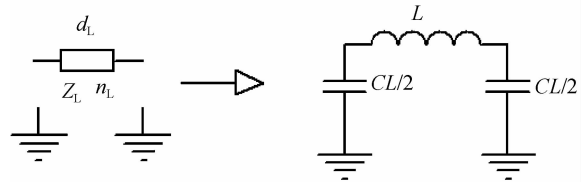
图4 \pi 型电路
