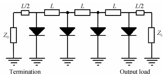
图 2 行波光二极管阵列结构
