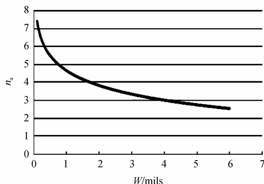
图6 n_a-W 曲线图
