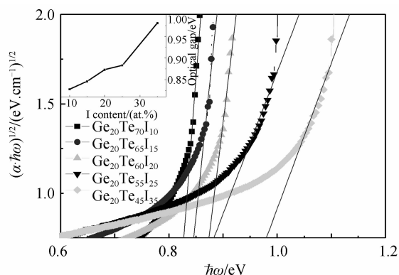
图5 图5玻璃样品 (\alpha \cdot \hbar\omega)^{1/2} 和 \hbar\omega 的关系(内插图为间接带隙 E_{\text{opt}} 与 I 含量的关系)
