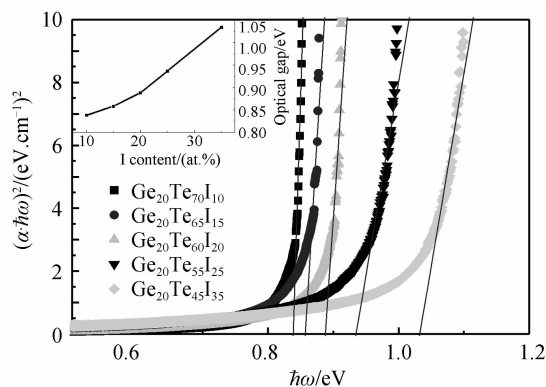
图4 玻璃样品 (\alpha \cdot \hbar\omega)^2 和 \hbar\omega 的关系(内插图为直接带隙 E_{\text{opt}} 与 I 含量的关系)
