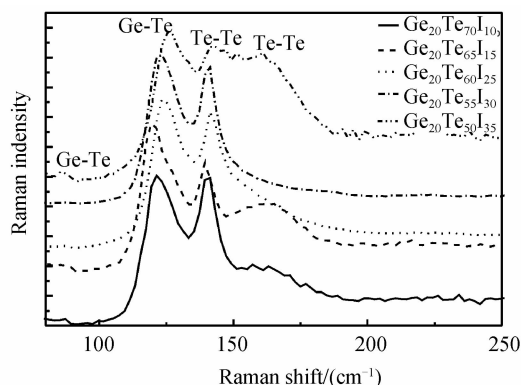
图6 玻璃样品的 Raman 光谱
