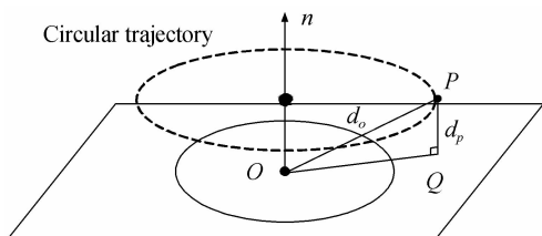
图 2 目标空间模型的两个约束 Fig. 2 Two constraints in object space model
