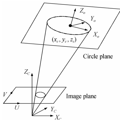
图 3 圆目标成像模型 Fig. 3 The imaging model of circular target
