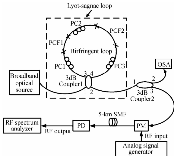
图 1 结构模型 Fig. 1 Schematic diagram
