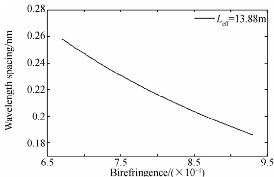
图 8 PCF 的有效长度为 13.88 m 时多波长光源的波长间隔和 PCF 双折射率的关系
