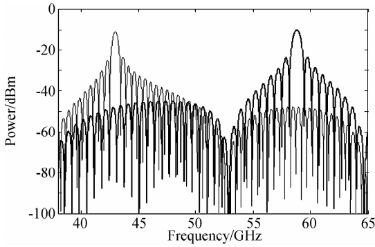
图9 MPF 的响应谱
