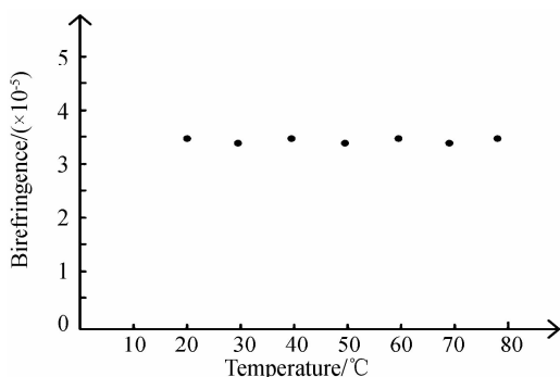
图 5 温度变化时光纤材料和空气对 PCF 双折射率的影响
