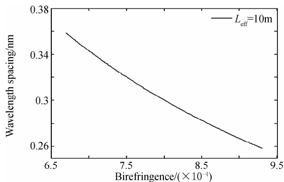
图 6 PCF 的有效长度为 10 m 时多波长光源的波长间隔和 PCF 双折射率的关系
