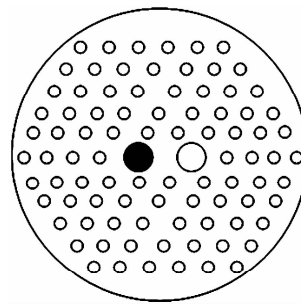
图 3 填充一个大孔后 PCF 的横截面图 Fig. 3 The cross-section of PCF after padding a big hole
