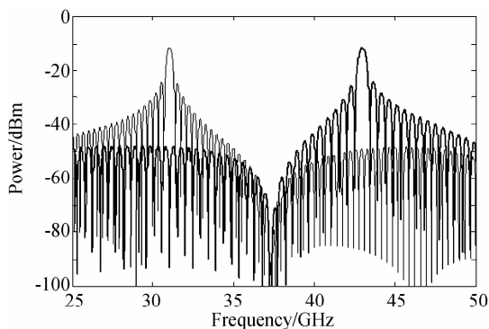
图 7 MPF 的响应谱
