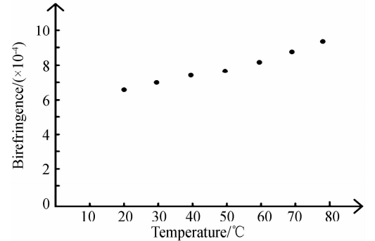
图 4 填充液体的温度与 PCF 双折射率的关系
