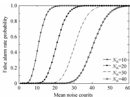
图 2 虚警率曲线
