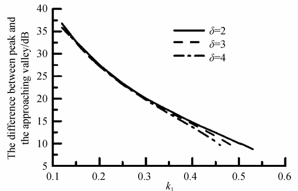
图 9 谐振点 D_{\max} 峰值和临近谷值的差值随外环强耦合系数 k_1 变化图
