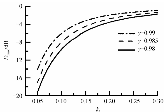
图 6 单环: 谐振点传输系数 D_{\max} 随场强耦合系数 k_1 变化关系图 Fig. 6 Single ring: The relationship of D_{\max} and k_1
