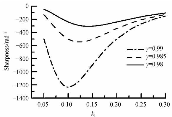
图 4 单环:尖锐度随场强耦合系数 k_1 的变化图
