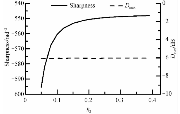
图 8 尖锐度 S_{\max,\varphi} 最大值和对应谐振点传输系数 D_{\max} 内环强耦合系数 k_2 与变化图
