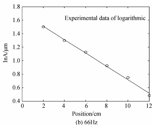
图 5 振幅对数的变化曲线 Fig. 5 The curved of the amplitude logarithm
