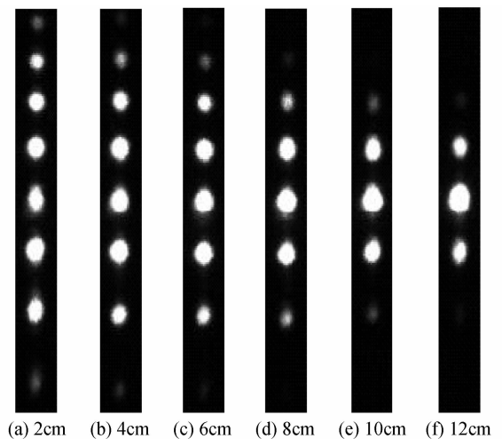
图 3 54 Hz 时在不同位置的衍射图样
