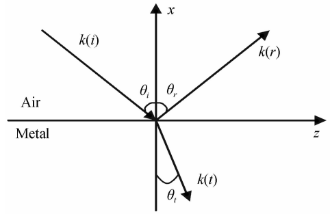
图 2 光在金属表面的反射和折射示意
