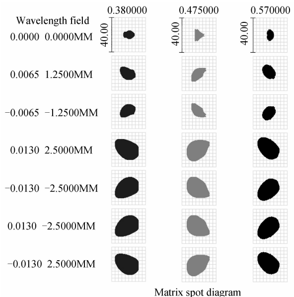
图 5 改进型 Czerny-Turner 光谱仪的点列图分布 Fig. 5 Spot diagram of modified Czerny-Turner spectrometer
