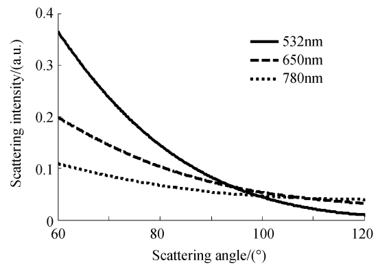
图 7 根据 Mie 散射理论计算的不同波长的散射光强与散射角度的关系曲线
