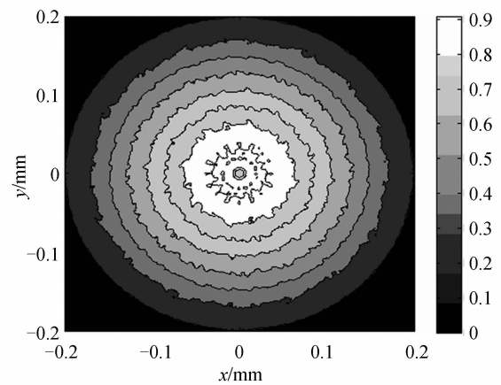
图 4 多光束叠加时光纤输出面的归一化光强分布
