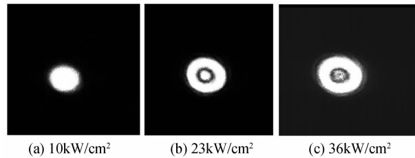
图 5 入射 532 nm 激光功率密度不同时远场衍射光斑图样
