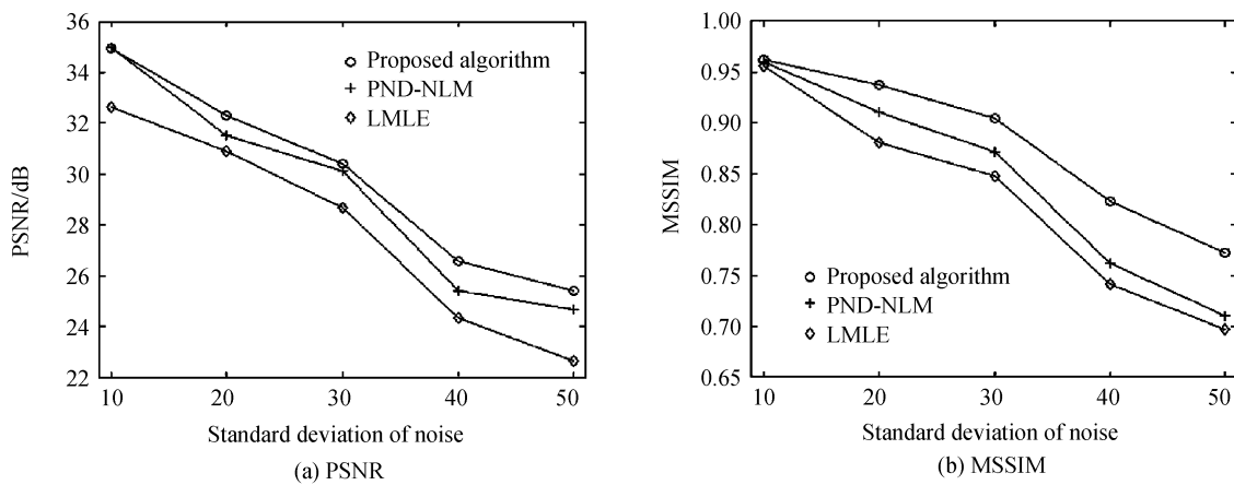
图 2 不同噪音等级本文算法、非局部均值算法和局部极大似然估计算法去噪结果 PSNR 和 MSSIM 比较
