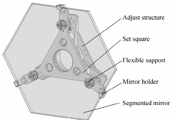
图 6 子镜室支撑模块 Fig. 6 Segment support module
