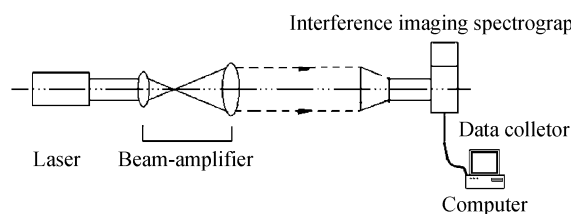
图 8 谱线位置与光谱分辨率检测装置
