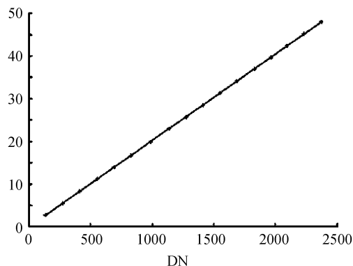
图 7 干涉成像光谱仪线性度
