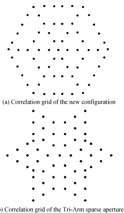
图 7 新型结构和三臂结构的相关点阵图 Fig. 7 Correlation grid of the new configuration and the Tri-Arm sparse aperture
