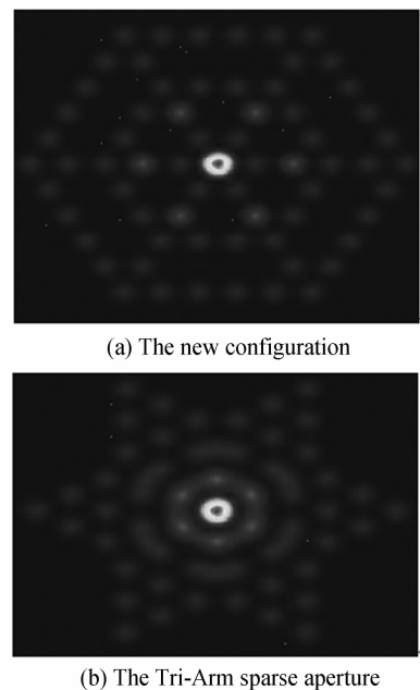
图 2 F=10\% 时新型结构和三臂结构的 MTF
