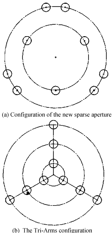
图 1 新型结构和三臂结构
