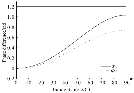
图5 不同入射角的相位差 \Phi_S 、 \Phi_P
