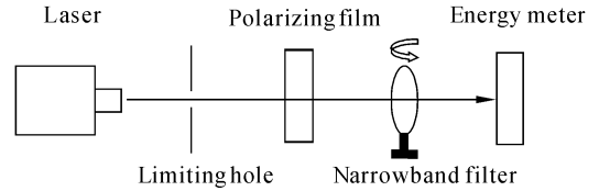
图6 滤光片透射率实验平台原理
