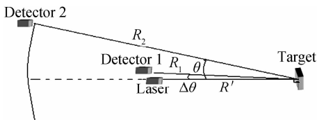
图 1 双光路探测
