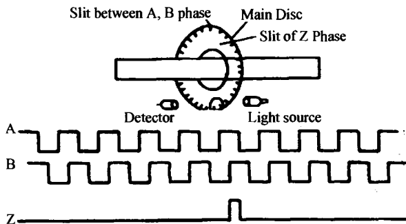
图 3 光电编码器结构示意图及输出波形 Fig. 3 Schematic diagram of structure of opto-electrical codifier and output pulse
