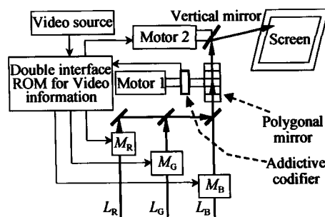
图 1 激光显示系统结构
