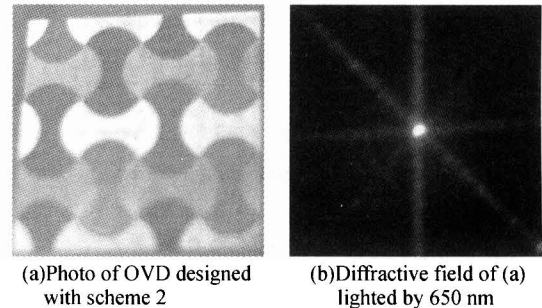
图 7 面阵 OVD 制作实例及衍射光场分布 Fig. 7 OVD sample designed with scheme 2
