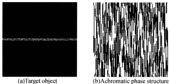
图 1 消色散位相结构的设计 Fig. 1 Designing of achromatic phase structure
