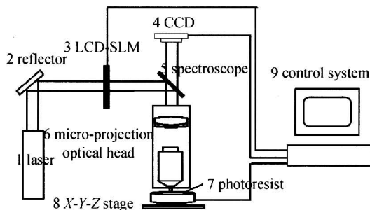
图 5 SVG-LDW04 系统结构图 Fig. 5 Illustration of SVG-LDW04
