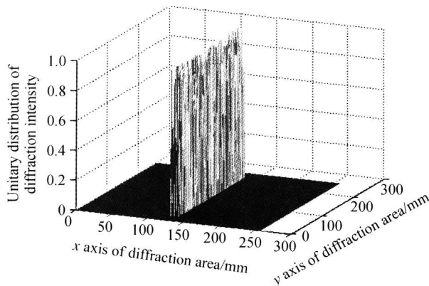
图 2 可见光区的衍射光强分布 Fig. 2 Diffractive wave distribution in visible spectrum
