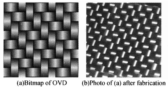
图 6 角度连续变化的点阵 OVD 实例 Fig. 6 Fabricated sample for a OVD with scheme 1
