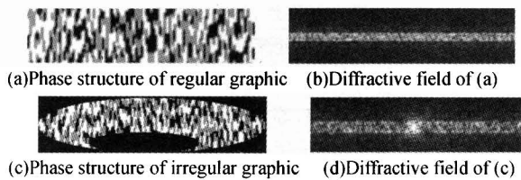
图 4 数据方案二 Fig. 4 Scheme 2
