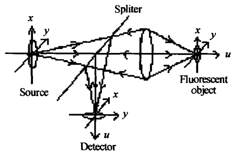
图 1 共焦显微镜的原理图
