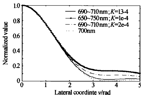
图 2 不同谱线范围、色散系数的横向分布 Fig. 2 Lateral distribution of fluorescent intensity
