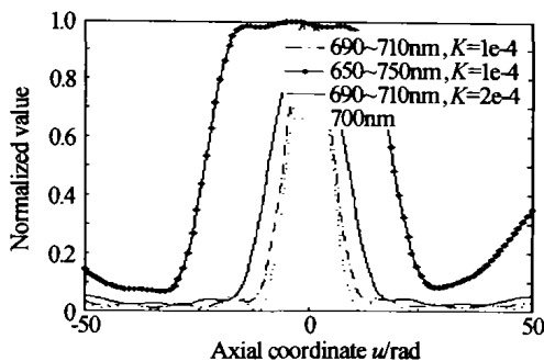
图 3 不同谱线范围、色散系数的纵向分布 Fig. 3 Axial distribution of fluorescent intensity
