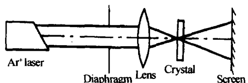
图 1 光损伤阈值强度测量装置 Fig. 1 Schematic diagram for photo damage threshold
