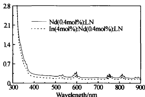
图 2 Nd:LiNbO 3 和 In:Nd:LiNbO 3 晶体的紫外-可见吸收光谱 Fig. 2 The Ultra-Visible absorption Spectrum of Nd:LiNbO 3 and In:Nd:LiNbO 3 crystal
