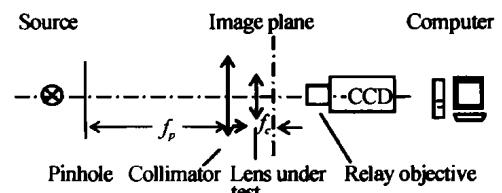
图 2 测试系统示意图
