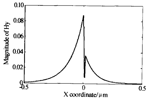
图 2 非对称型表面模的场分布
