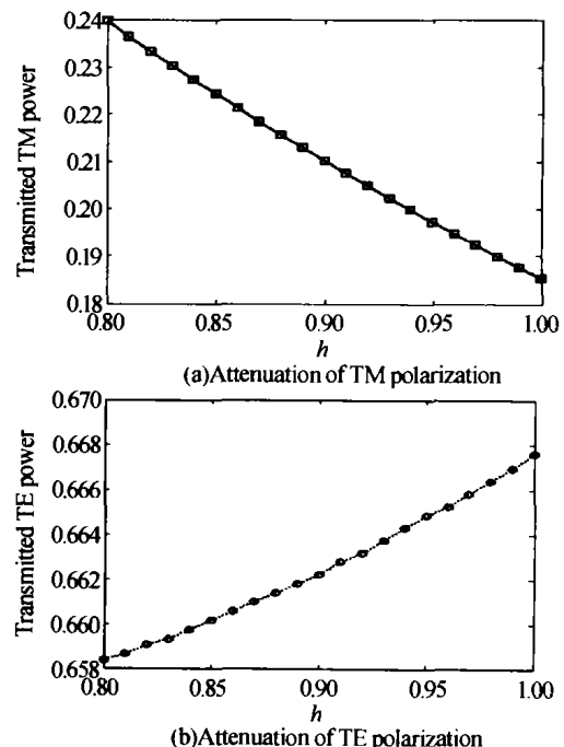
图 6 接受端光功率随氢气浓度的变化 Fig. 6 Transmitted power versus hydrogen concentration
