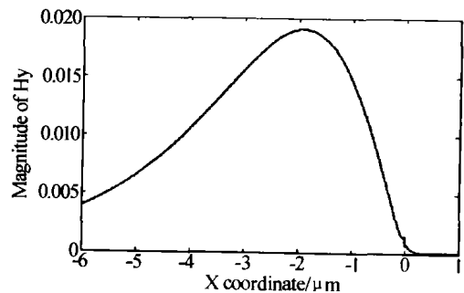
图 3 导模的场分布
