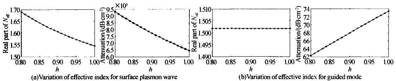
图 4 不同氢气浓度时有效折射率的变化 Fig. 4 Effective index verse concentration of hydrogen
