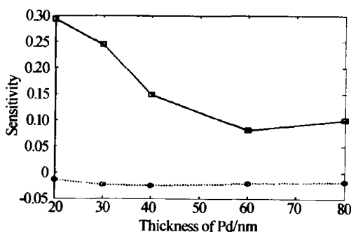
图 5 不同厚度 Pd 膜的灵敏度 Fig. 5 Sensitivity of hydrogen sensor for different Pd layer thickness
