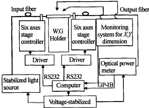
图1 系统结构
