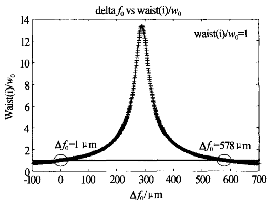
图 4 束腰半径比 vs 离焦距离
