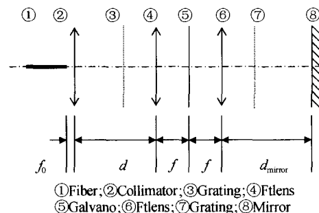
图 2 RSOD 展开图
