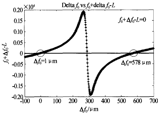
图 3 离焦距离 vs 束腰距离差
