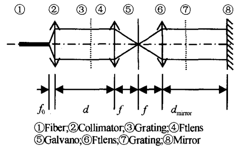
图 5 RSOD 中高斯光束分布图
