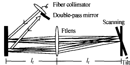
图 1 双光程快速扫描光学延迟线
