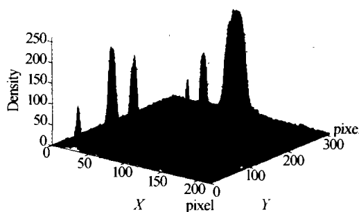
图5 光斑的强度分布 ( V_a = 3700 \text{ V} )
