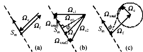
图 1 一阶后补偿的两种方式
