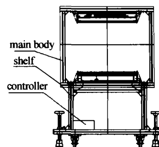
图2 光幕靶系统图 Fig. 2 Light screen system
