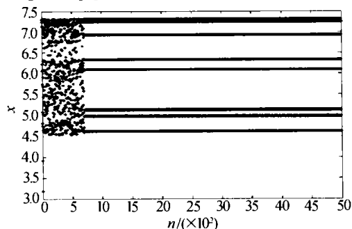
图8 8p周期轨道( A=0.22, B=0.66 )
