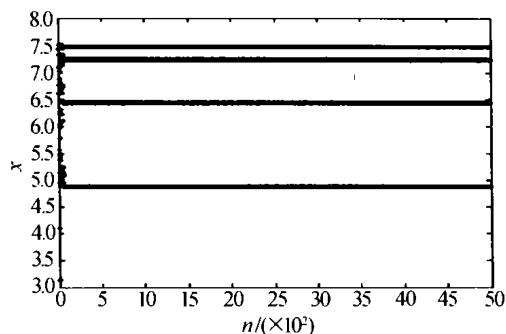
图5 原系统4p周期轨道的稳定( A=0.51 )
