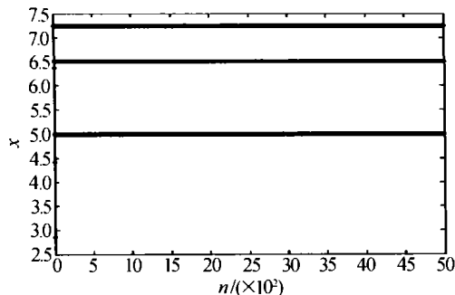
图6 3p周期轨道( A=0.66, B=0.89 )
