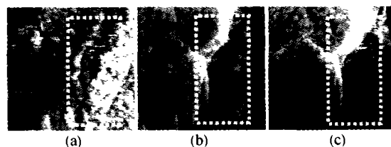
图 7 铁腐蚀过程的液相型 AFM 扫描图像, 时间间隔 2 min, 扫描范围 1500\text{ nm} \times 1500\text{ nm}
