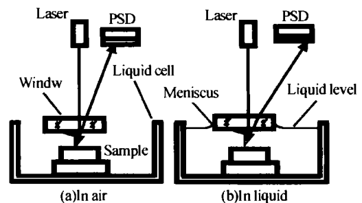
图 1 AFM 光路图
