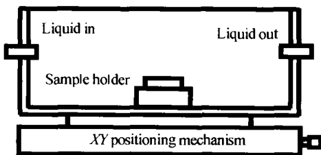
图3 液体池 Fig. 3 Liquid cell
