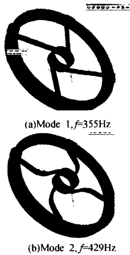
图 6 结构 3 的前二阶模态 Fig. 6 The first two modes of structure 3
