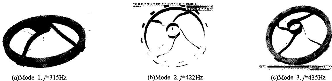
图 9 叶片宽度 3 mm 模态 Fig. 9 The modes of 3 mm plate
