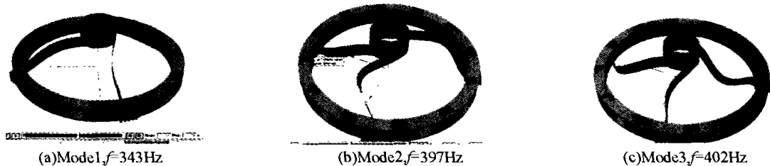
图 8 5 mm 叶片宽度的模态 Fig. 8 The modes of 5 mm plate
