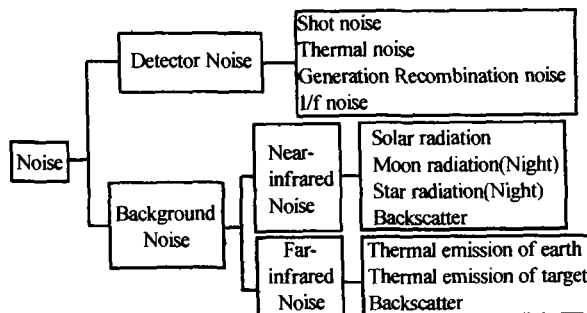
图1 噪声模型构成框架图 Fig. 1 Sketch of noise model
